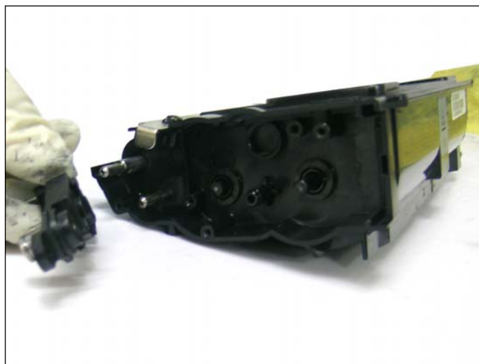
16. Soporte del rodillo de revelación extraído.
