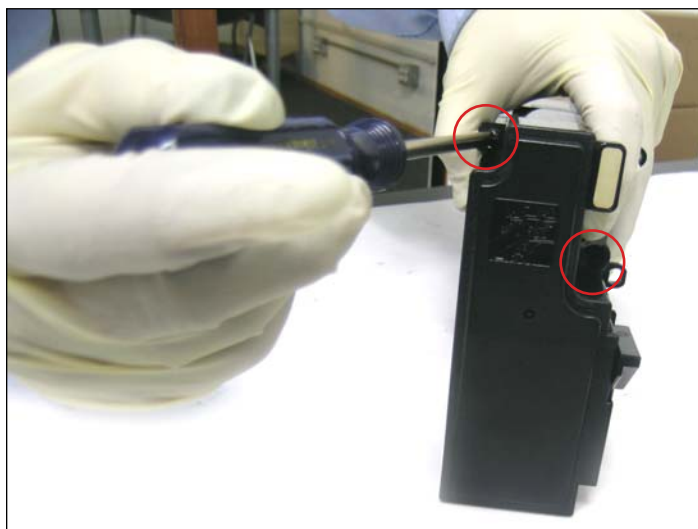
1. Retirar los dos tornillos que unen el depósito de desperdicios con el resto del cartucho.
